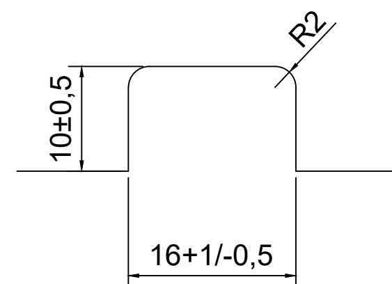
STOPPER GROOVE
