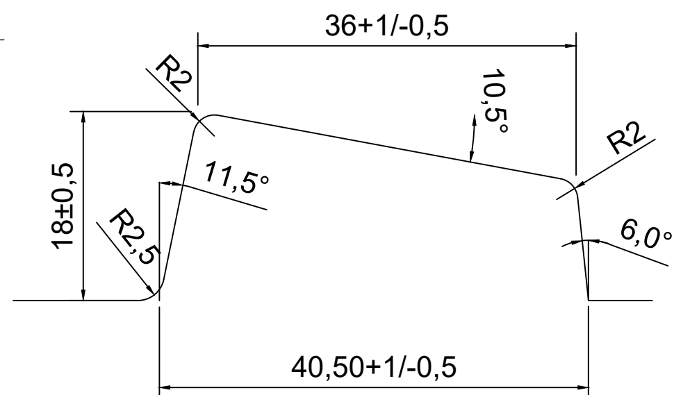
REKA GROOVE TYPE 3
