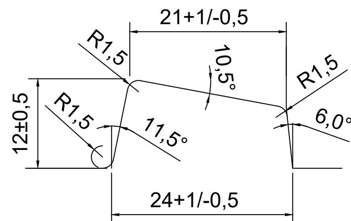
REKA GROOVE TYPE 1
