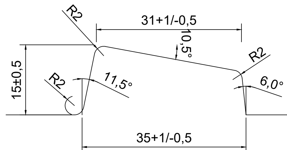
REKA GROOVE TYPE 2
